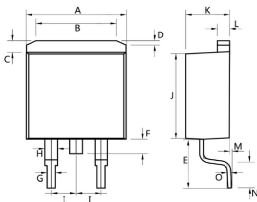
TO-263-2L
